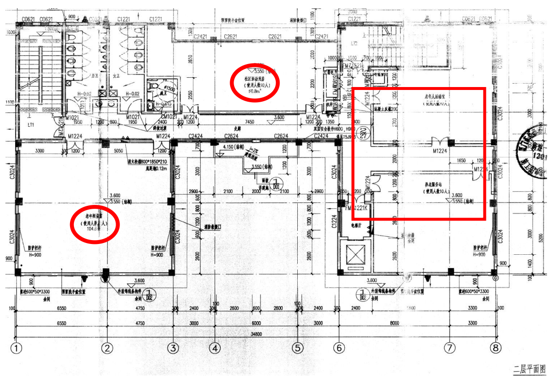
二层审批图纸:
