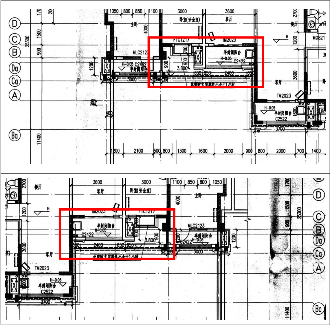
审批建施图（二层）：
